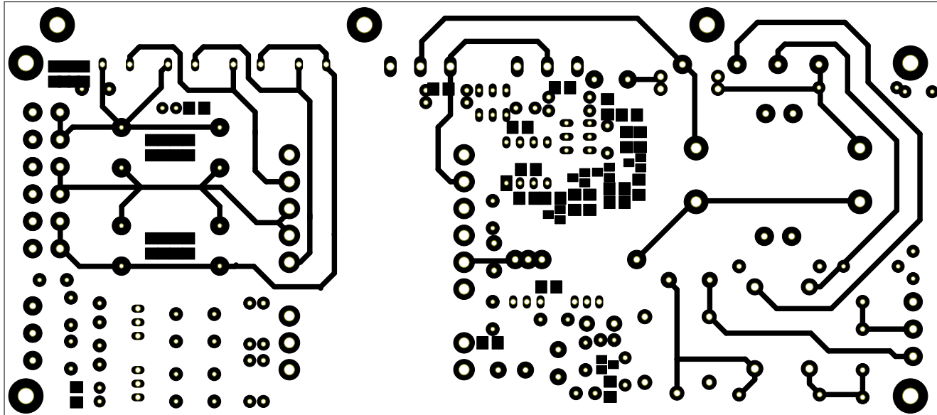
bottom mask
